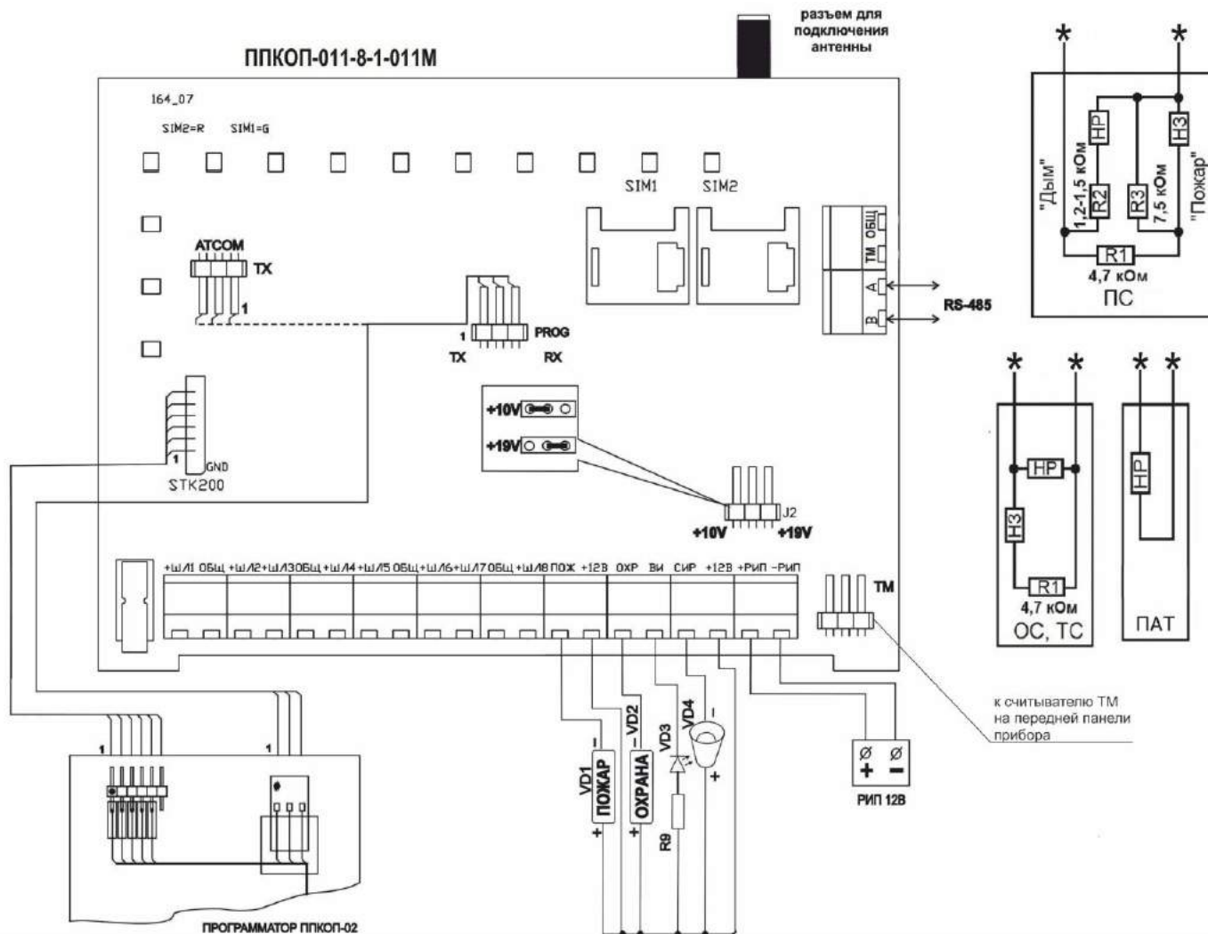
Рисунок 2. Схема подключения прибора
