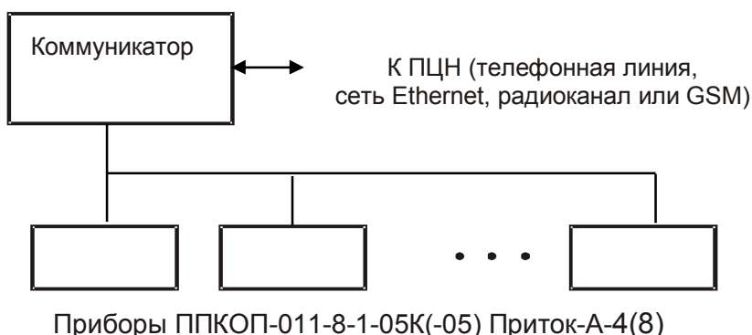
Рисунок 1. Схема связи приборов с коммуникатором.
