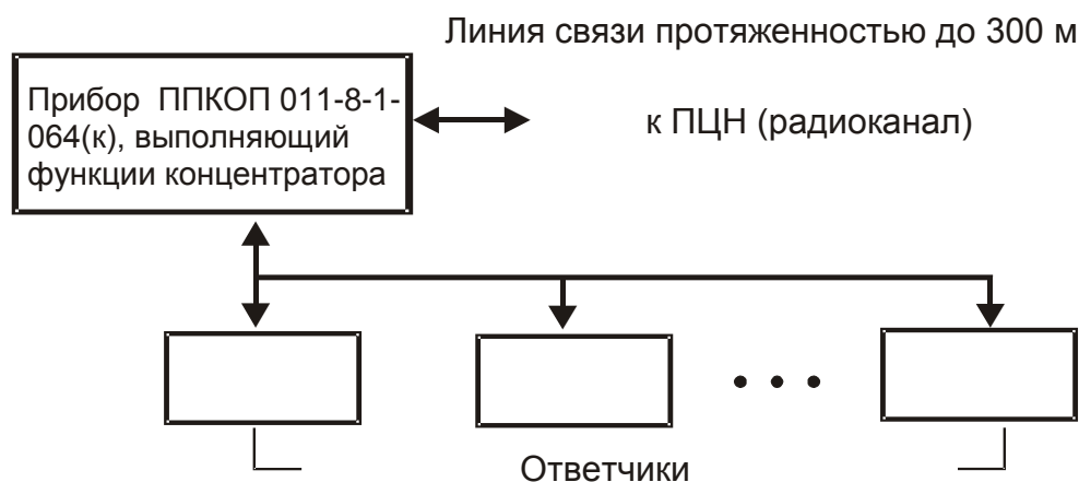
Рисунок 1. Схема связи ответчиков с прибором
