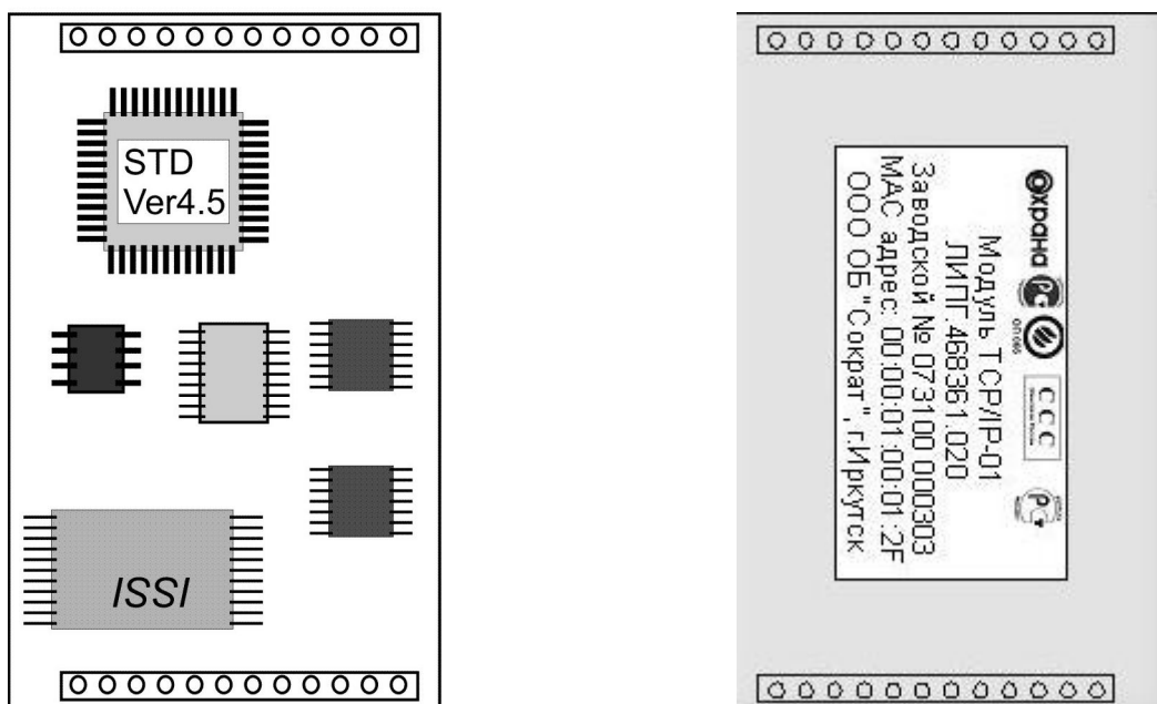
Модуль TCP/IP (код:0730XX) (вид снизу)
