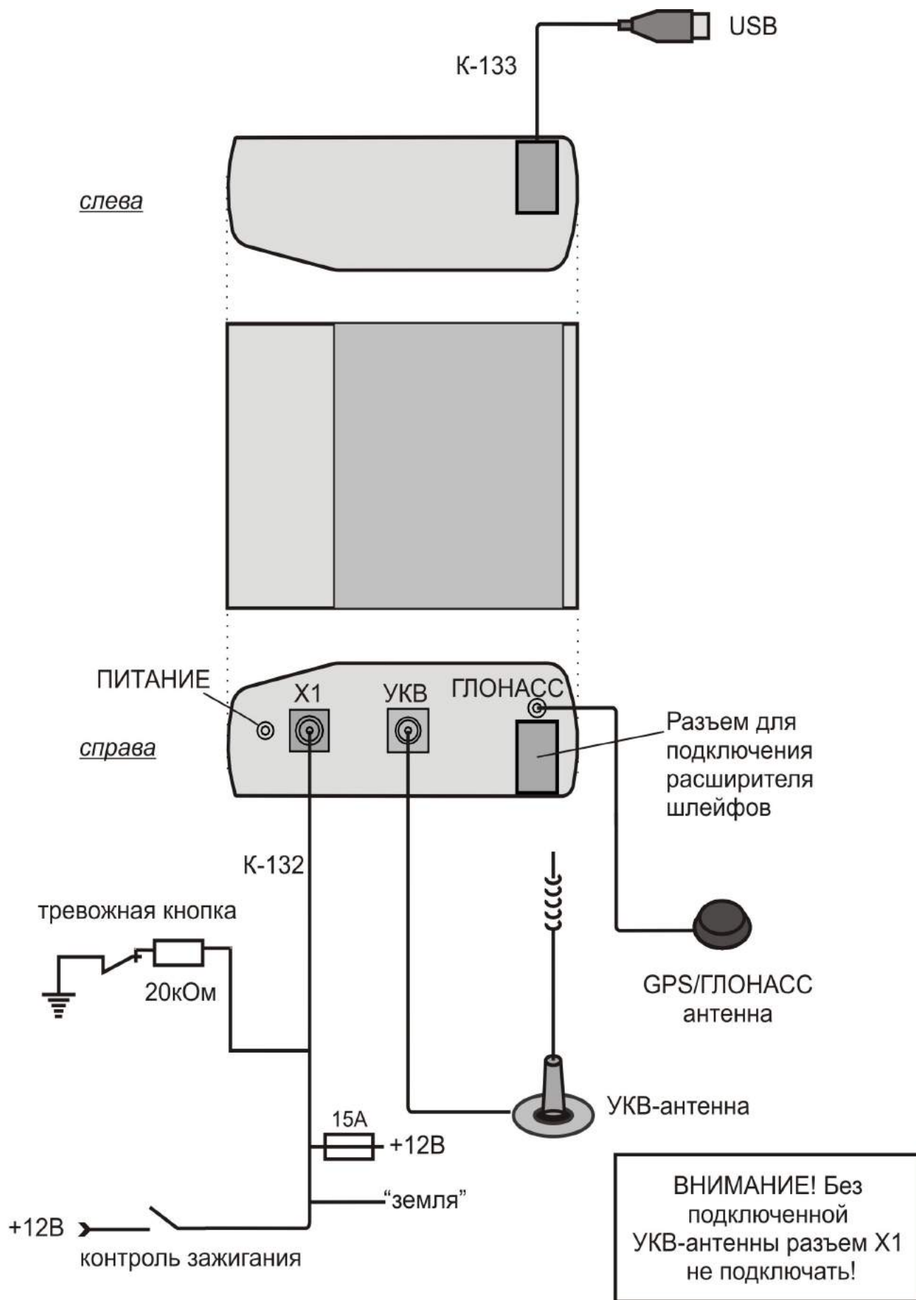
Рисунок 1: Монтажная схема Приток БК-011(-021)
