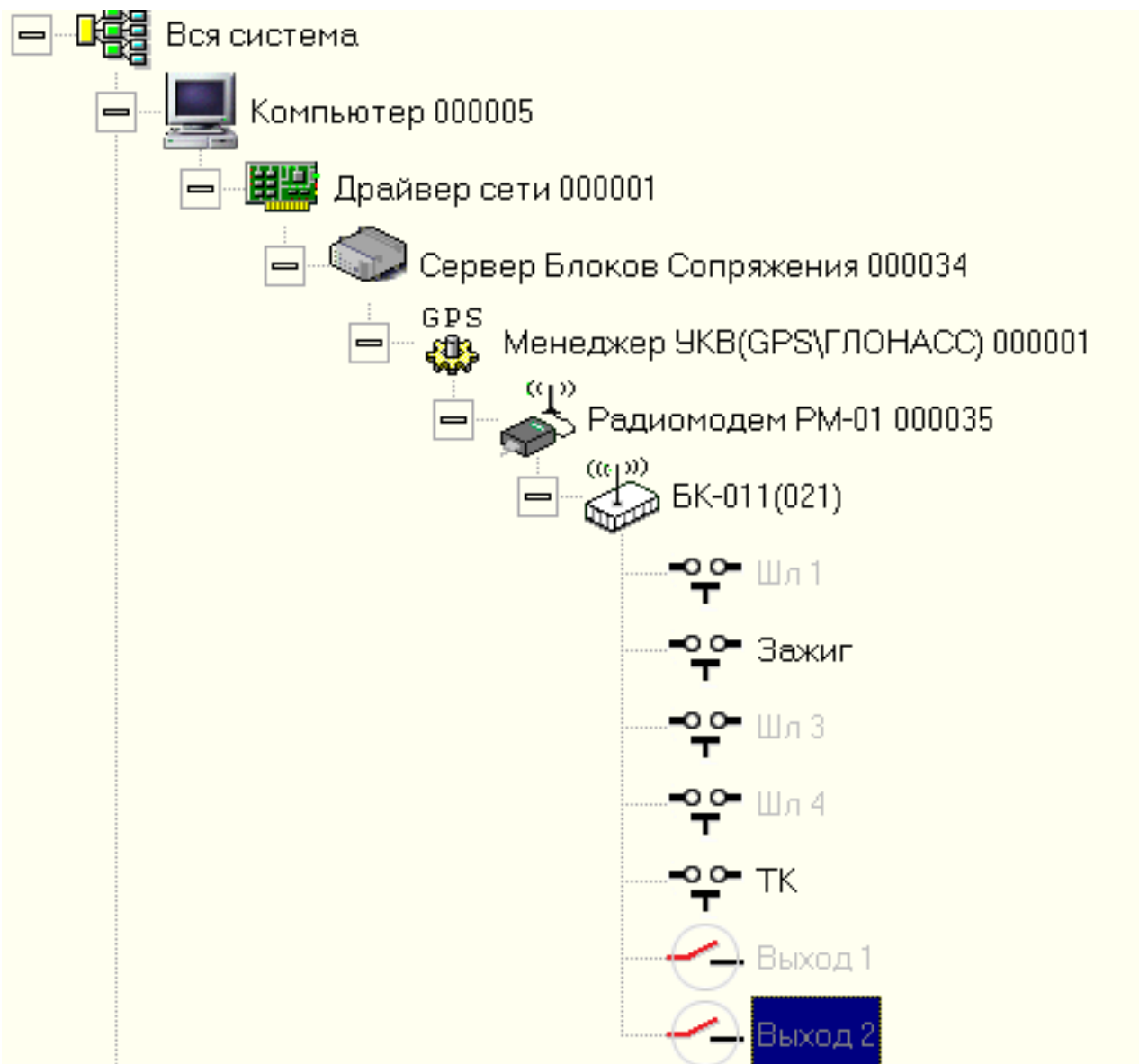
Рисунок 2: Описание Приток БК-011(-021)
