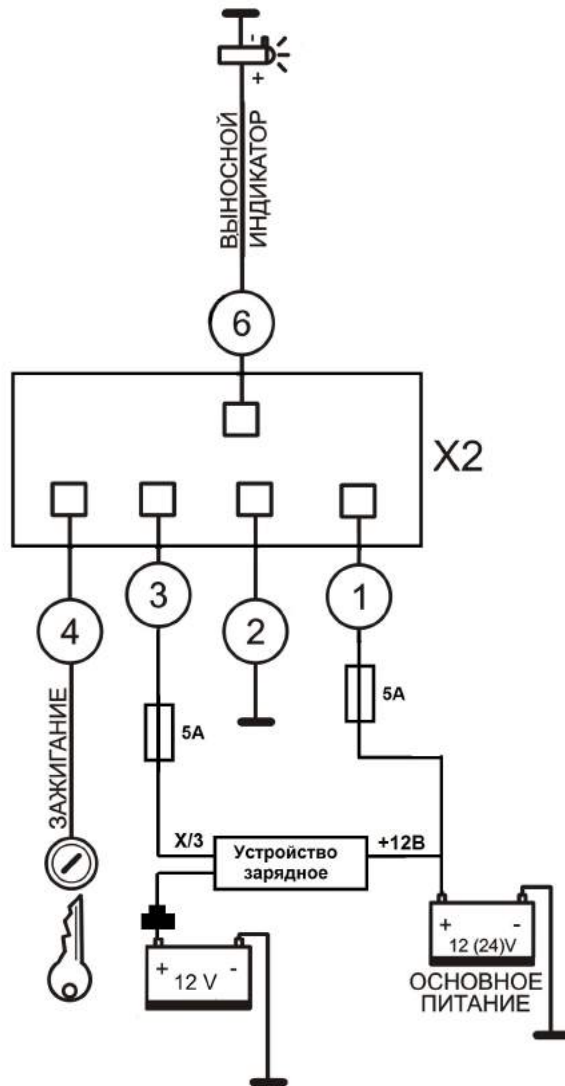
Рисунок 5 – Схема подключения с зарядным устройством
