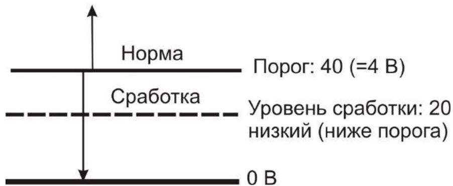
Рисунок 8 - Низкий уровень сработки входа «Дверь».
