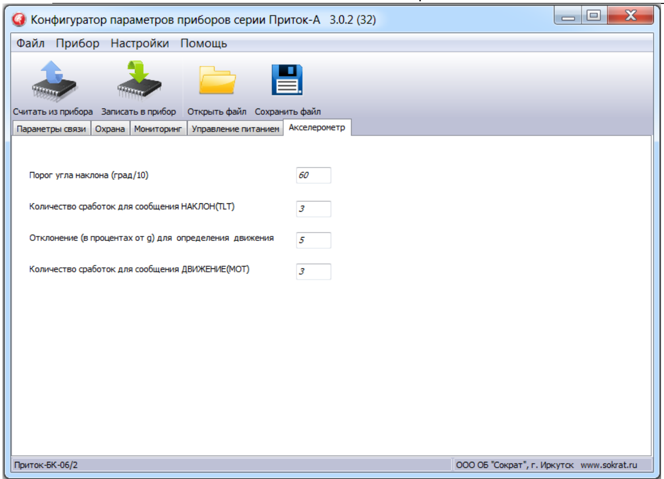
Рисунок 6 – Вкладка «Акселерометр»
