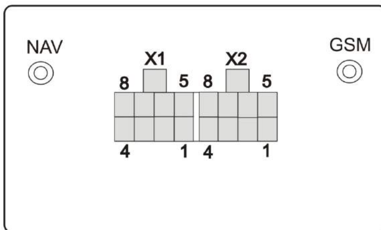
Рисунок 2 - Тыльная сторона
