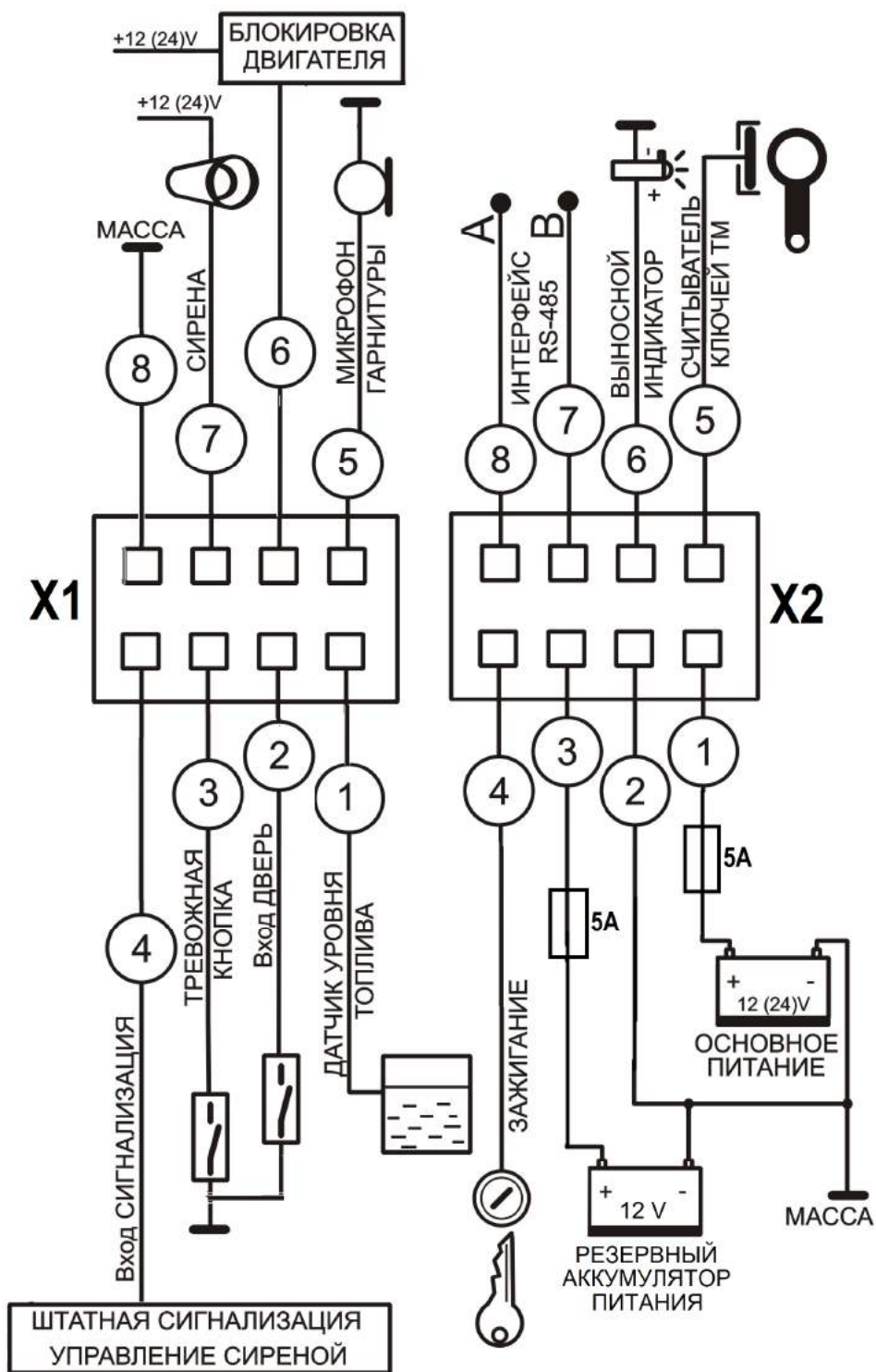
Рисунок 3 - Схема подключения БК-06
