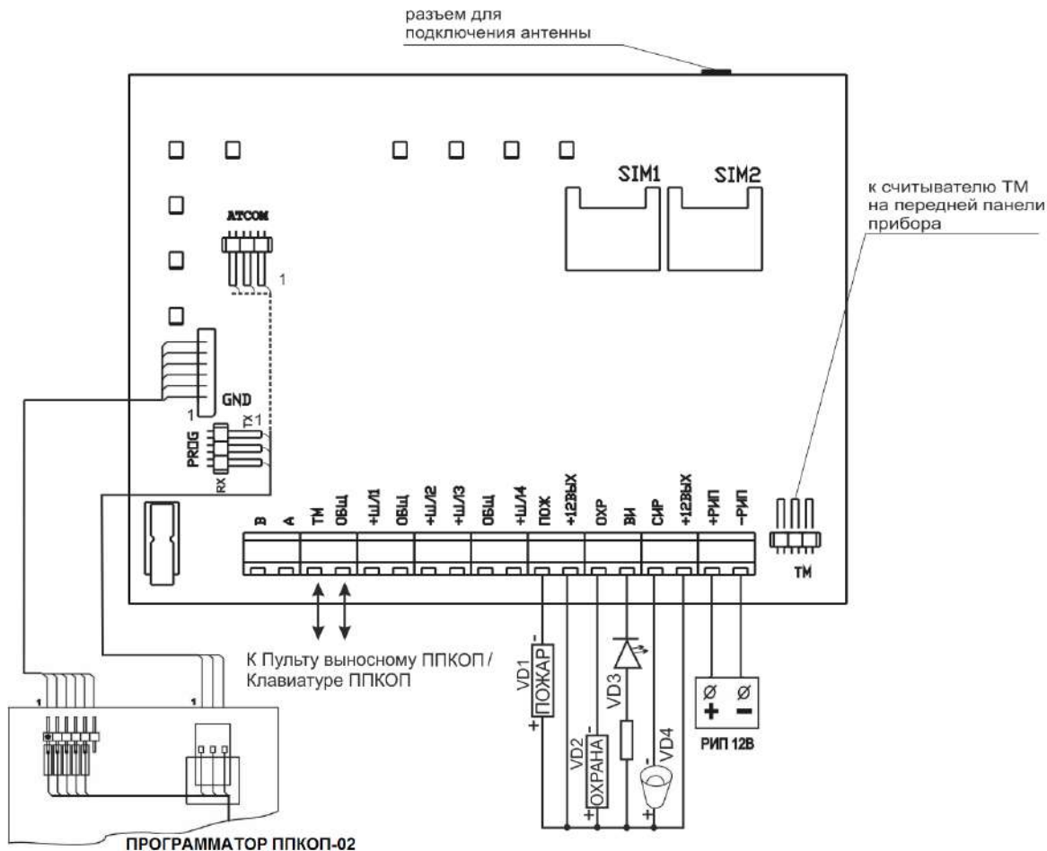
Рисунок 2. Схема подключения прибора
