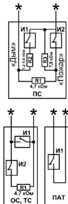
Рисунок 3. Схема организации ШС
