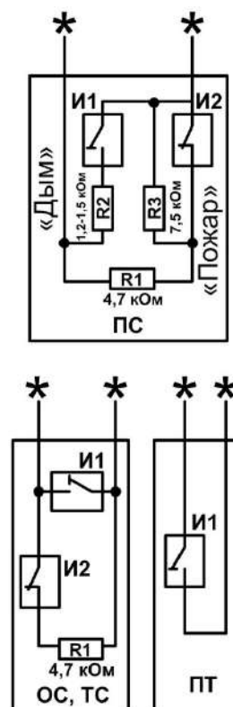
Рисунок 7 – Схема организации ШС
