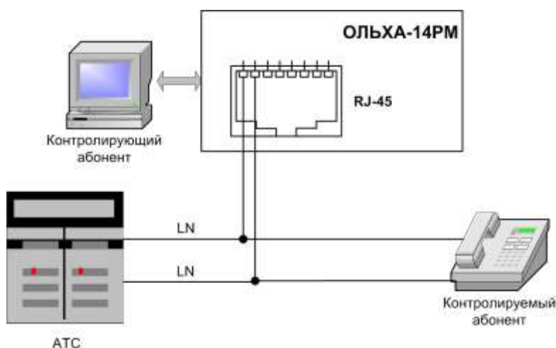
Рис.9 Параллельное подключение
