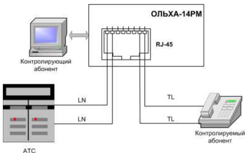
Рис.8 Подключение в разрыв
