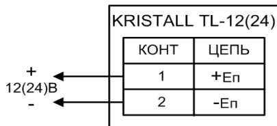
Рис.1 Схема подключения.
