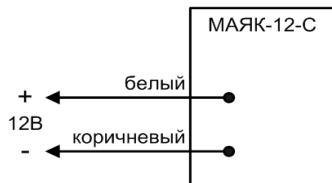
Рис.1 Схема подключения.
