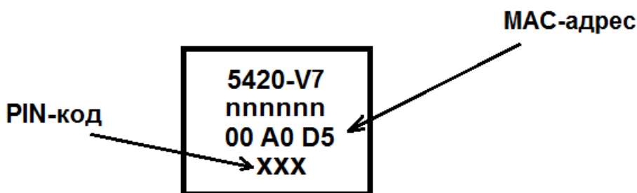
Рисунок 4. Шильдик на плате модуля
